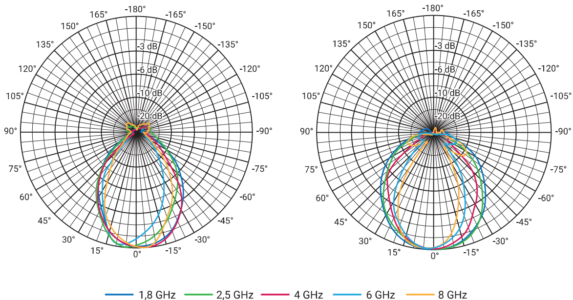
Horizontal und Vertical Pattern HyperLOG® 30 X Series
