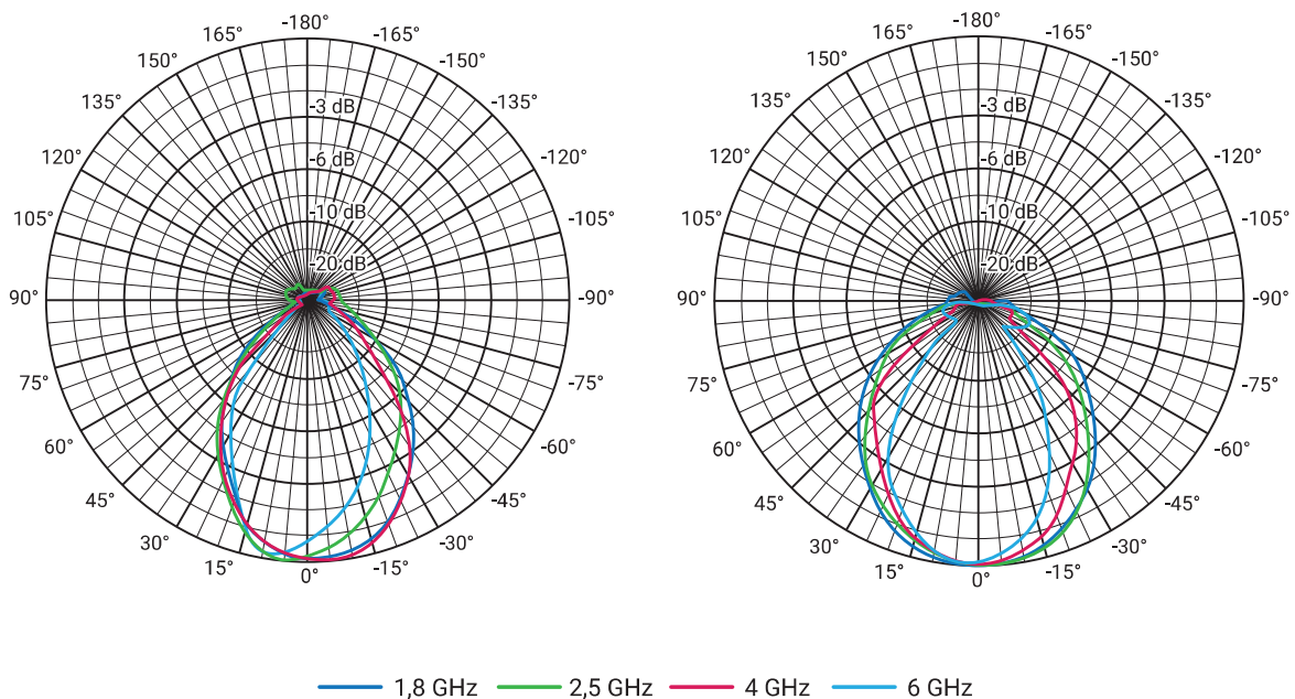
Horizontal und Vertical Pattern HyperLOG® 70 X Series
